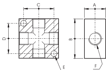
TEE CROSS MANIFOLD / REPARTITEUR EN CROIX / RIPARTITORE A CROCE
