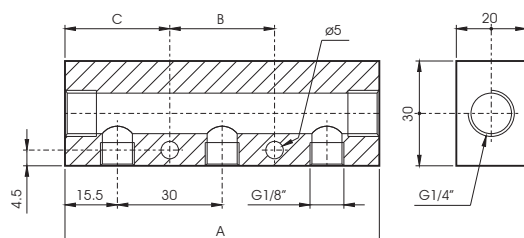
SINGLE MANIFOLD 1/4 - 1/8 / COLLECTEUR 1/4 - 1/8 / RIPARTITORE SINGOLO 1/4 - 1/8
