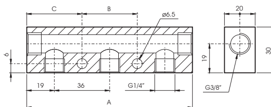
SINGLE MANIFOLD 3/8 - 1/4 / COLLECTEUR DOUBLE 3/8 - 1/4 / RIPARTITORE SINGOLO 3/8 - 1/4
