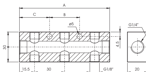
DOUBLE MANIFOLD 1/4 - 1/8 / COLLECTEUR DOUBLE 1/4 - 1/8 / RIPARTITORE DOPPIO 1/4 - 1/8
